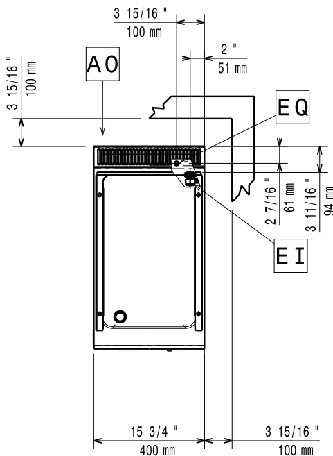
Boven aanzicht
